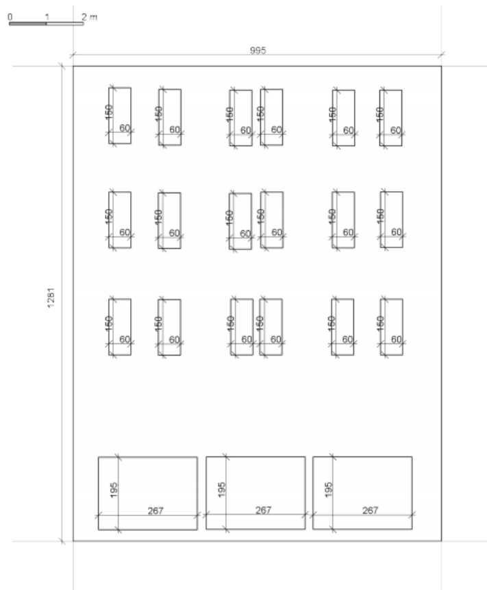
Ausschnitt vom automatisch generierten Fassadenplan
