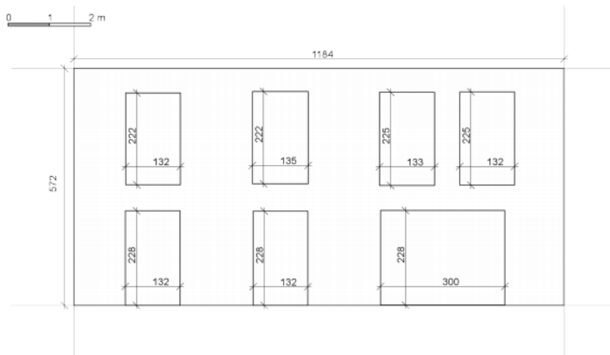
Ausschnitt vom automatisch generierten Fassadenplan
